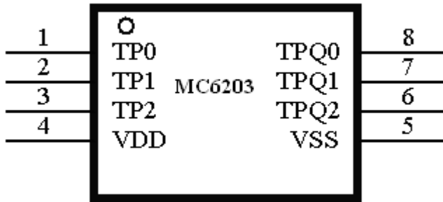
MC6203 SOP8 脚位图:
